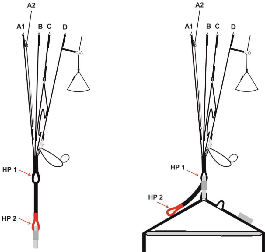
Fig. 7: TWIN 5 S vario-riser
